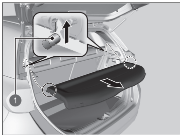
1 Haltestrebe
