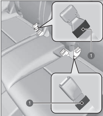
1 Schlaufe
