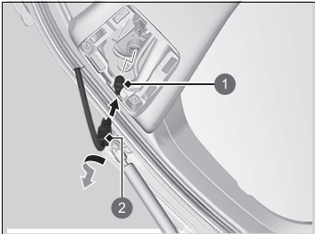
1 Glühlampe 2 Fassung
